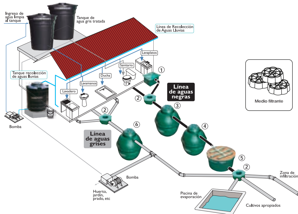
⑥ Tanque para tratamiento de aguas grises 250 L / 500 L / 1000 L / 2000 L
